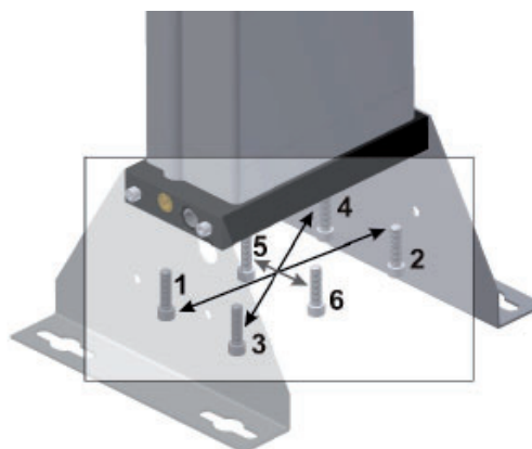
Poprawny montaż płyty zaworów elektromagnetycznych
